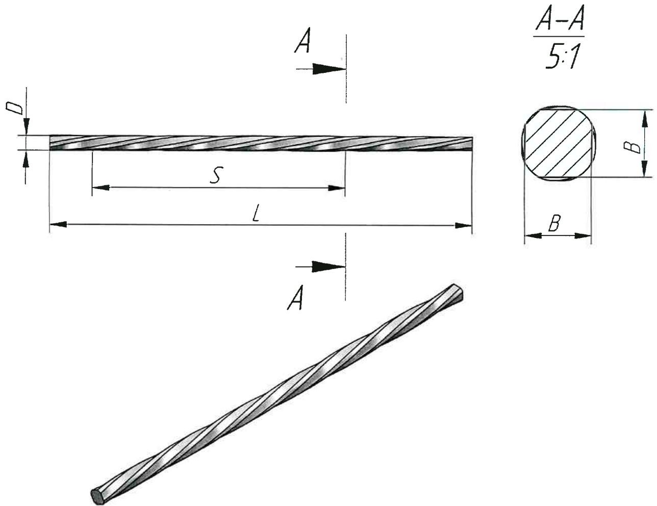
Рис. 1 Проволока винтовая.
